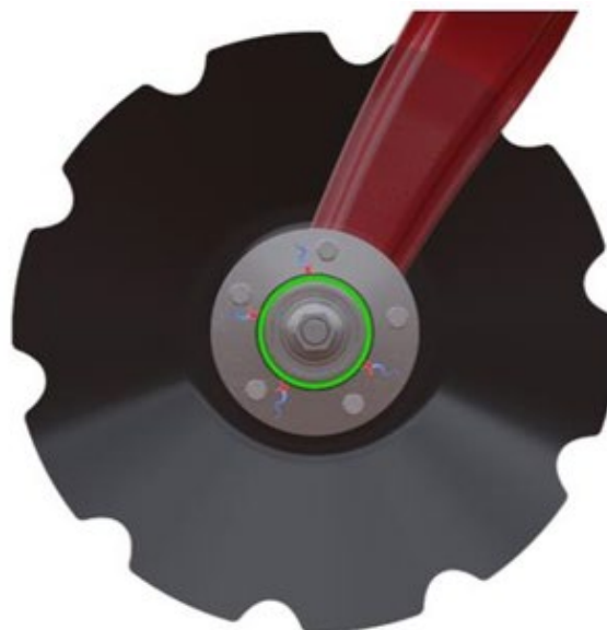
Eredeti - a csapágy védett
